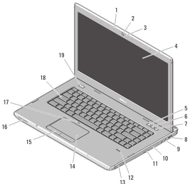
Rysunek 5. Vostro 3550 — widok z przodu
